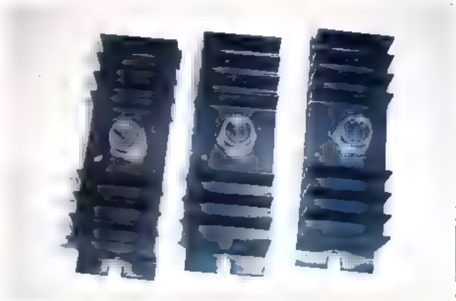
Foto 3: Helaas nauwelijks nog te krijgen: 25 watt zenerdiodes op koelplaat.
